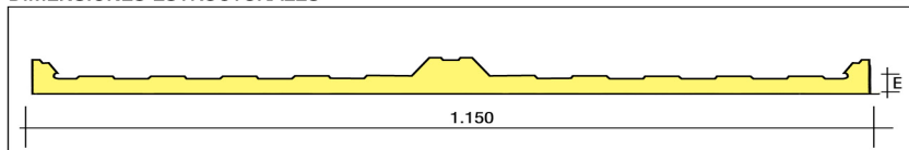
DIMENSIONES ESTRUCTURALES
