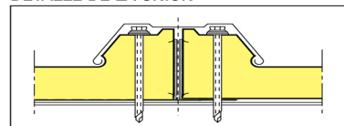
DETALLE DE LA UNIÓN
